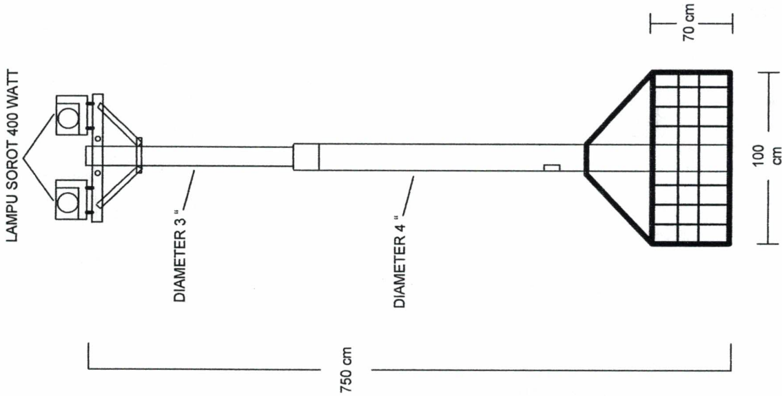
TIANG UNTUK LAMPU SOROT (NON PERMANEN)
