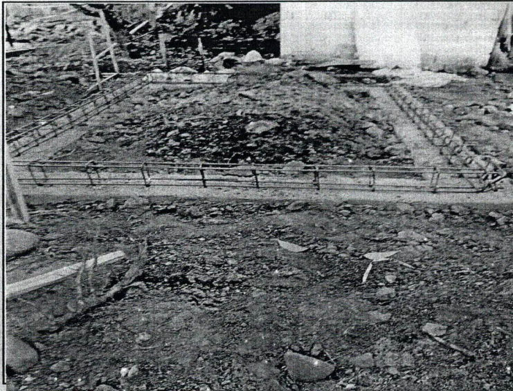
PEMBESIAN SLOF
