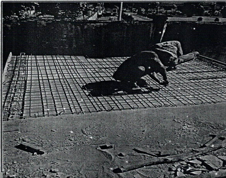
PEMBESIAN ATAP
