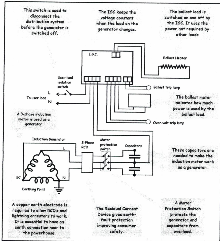
Gambar II.2 Koneksi Generator dan kontroler
