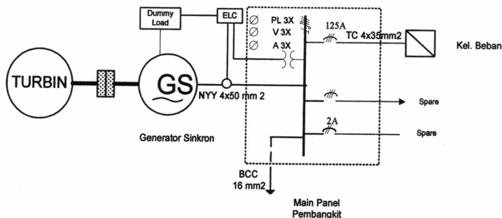
Gambar 4.2 Generator Sinkron dan Sistem Kontrolnya (ELC)
