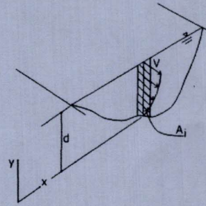
Gambar 4.1. Distribusi kecepatan air pada penampang sungai
