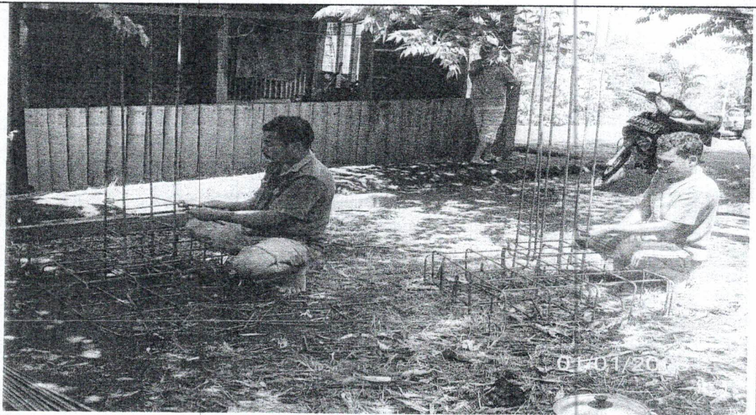
Gambar: Pembesian untuk Pondasi Plat
