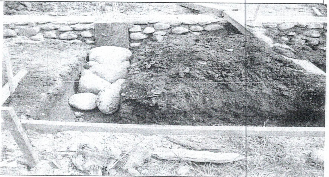
Gambar: Pembesian untuk Pondasi Plat
